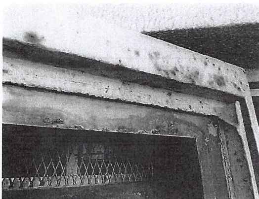
PS扉内部 錆発生箇所
