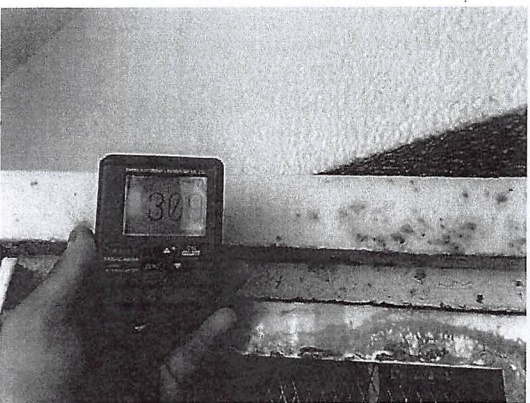
PS扉内部 錆発生箇所 膜厚確認
